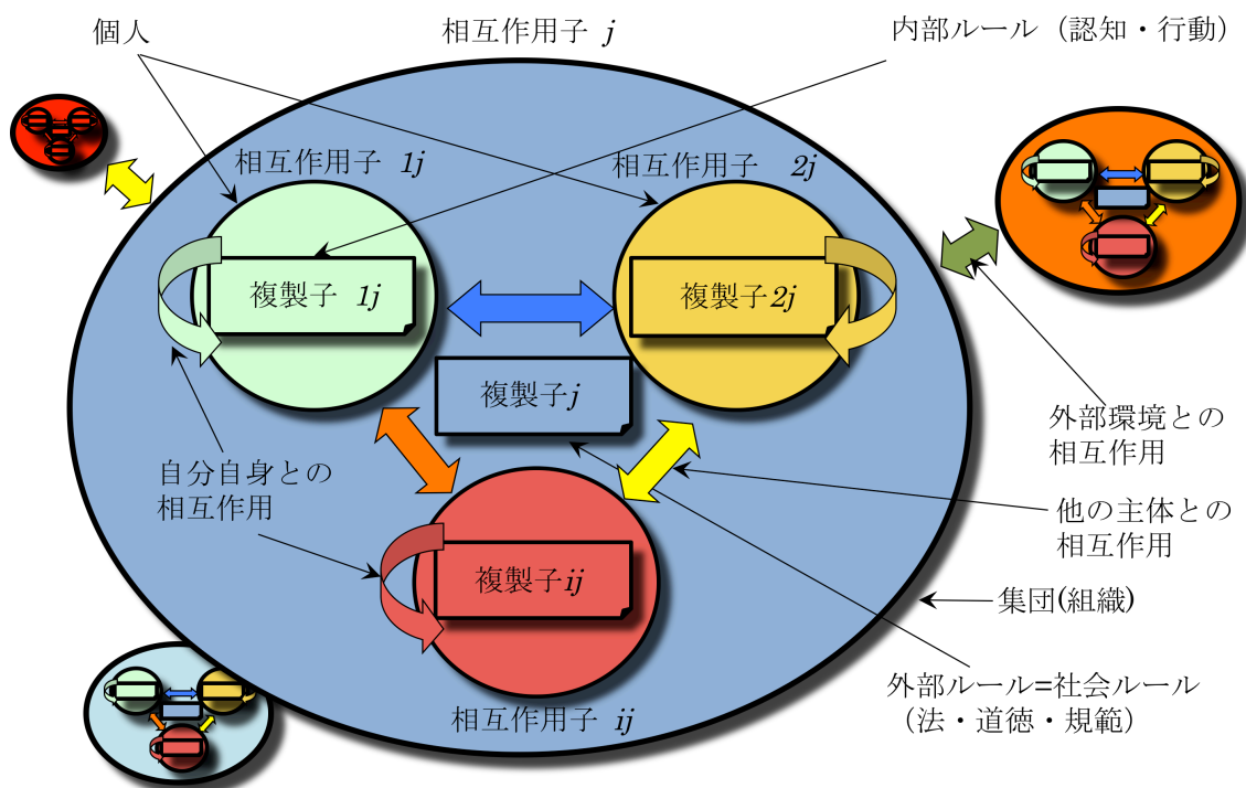
図 1 複製子と相互作用子の入れ子構造
